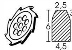
Carbide blade Ø 110 x 4.5 mm
