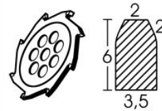
Carbide blade Ø 110 x 3.5 mm
